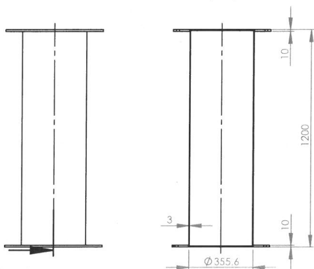
PRZEKRÓJ A-A
